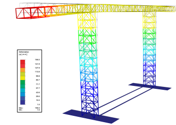
Deformation max. Wind, längs Verformungen (10-fach überzeichnet)
