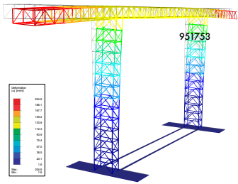
Deformation max. Wind, quer Verformungen (10-fach überzeichnet)
