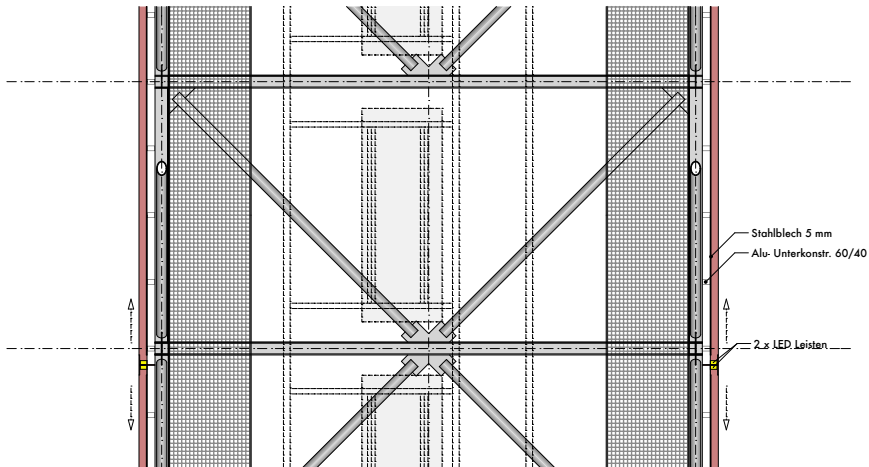
Grundriss Ausschnitt M1:20
