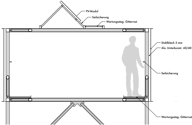
Detailschnitt M1:20
