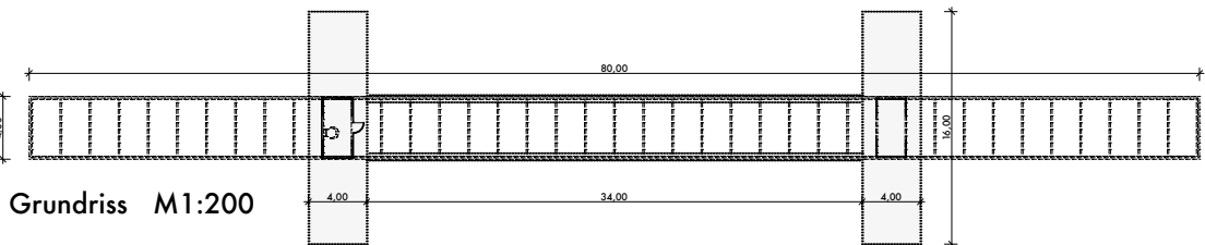
Draufsicht M1:200
