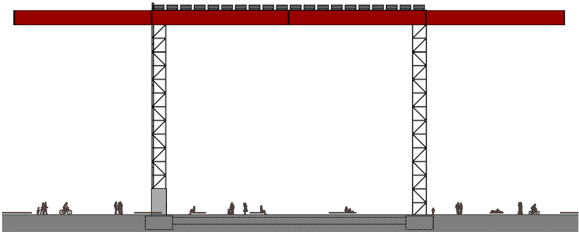
Ansicht M1:200
