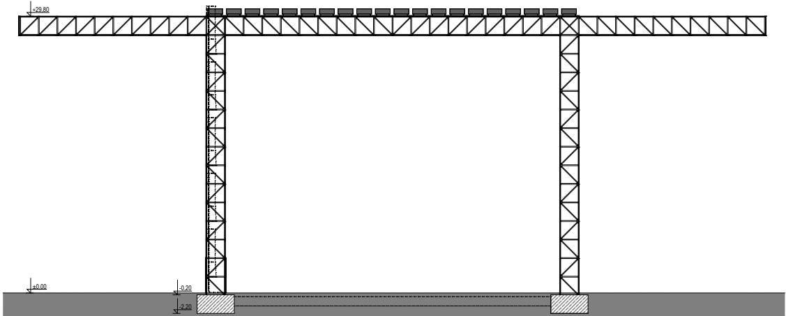
Längsschnitt M1:200
